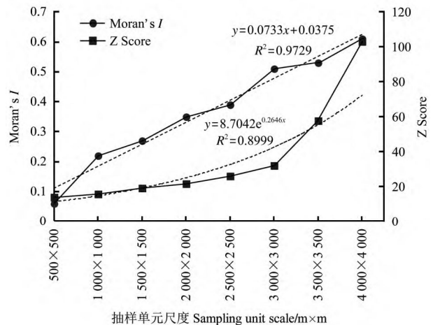
图3 全局空间自相关指数 Moran's I 随抽样单元尺度的变化情况
