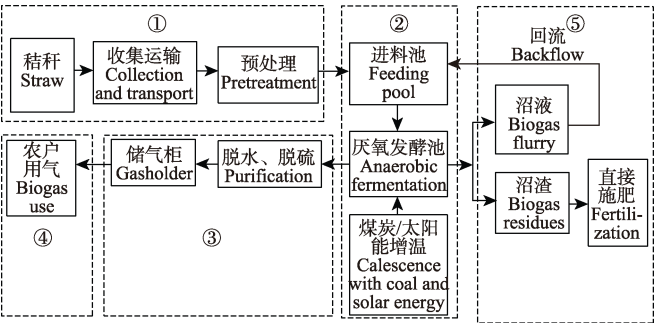
①秸秆收集与处理子系统 ②厌氧发酵子系统 ③净化贮存子系统 ④管网供气子系统 ⑤沼液利用子系统 ①Straw collection and treatment subsystem ②Anaerobic fermentation subsystem ③Purification storage subsystem ④Pipe network gas supply subsystem ⑤Biogas utilization subsystem
