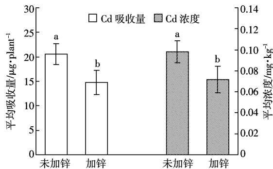
图 2 加锌与未加锌处理条件下,豇豆豆角中的平均 Cd 浓度及平均吸收量
